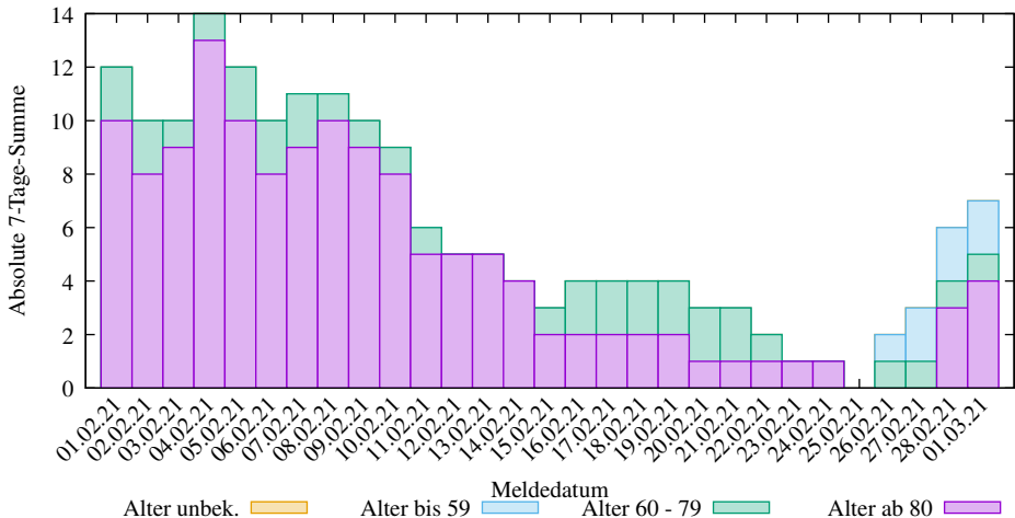
Abs. 7-Tage-Summen der neuen COVID-19 Verstorbenen in LK Offenbach (2025-03-09/2102, D. Lippold, https://covid19-de-stats.sourceforge.io/ Lizenz: CC BY-ND 4.0, Daten: Robert Koch-Institut (RKI), dl-de/by-2-0)
