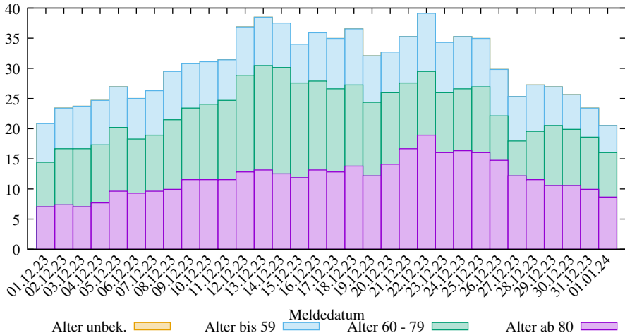
Rel. 7-Tage-Summe der neuen COVID-19 Infizierten in SK Mannheim (2025-03-09/2312, D. Lippold, https://covid19-de-stats.sourceforge.io/ Lizenz: CC BY-ND 4.0, Daten: Robert Koch-Institut (RKI), dl-de/by-2-0)
