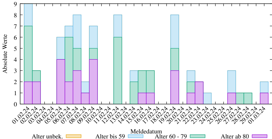
Einzelwerte der neuen COVID-19 Infizierten in SK Mannheim (2025-03-09/2402, D. Lippold, https://covid19-de-stats.sourceforge.io/ Lizenz: CC BY-ND 4.0, Daten: Robert Koch-Institut (RKI), dl-de/by-2-0)
