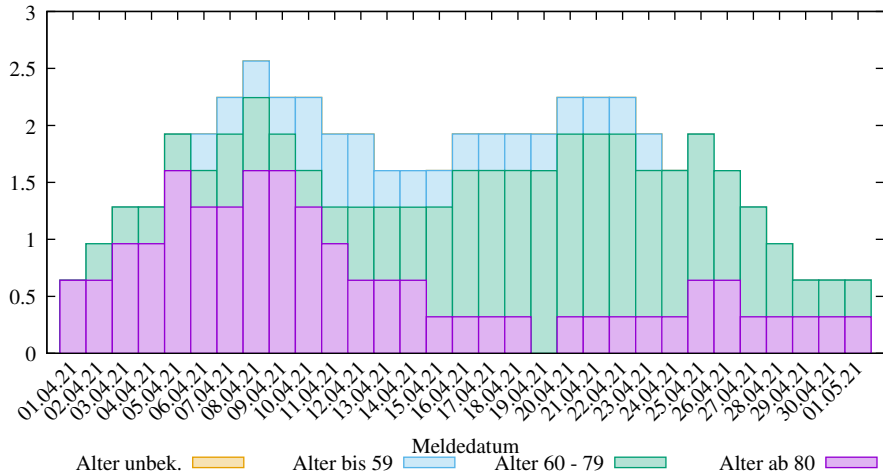
Rel. 7-Tage-Summe der neuen COVID-19 Verstorbenen in SK Mannheim (2025-03-09/2104, D. Lippold, https://covid19-de-stats.sourceforge.io/ ) Lizenz: CC BY-ND 4.0, Daten: Robert Koch-Institut (RKI), dl-de/by-2-0)
