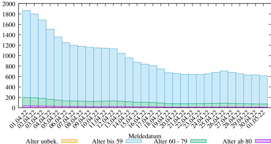
Rel. 7-Tage-Summe der neuen COVID-19 Infizierten in SK München (2025-07-06/2204, D. Lippold, https://covid19-de-stats.sourceforge.io/ Lizenz: CC BY-ND 4.0, Daten: Robert Koch-Institut (RKI), dl-de/by-2-0)
