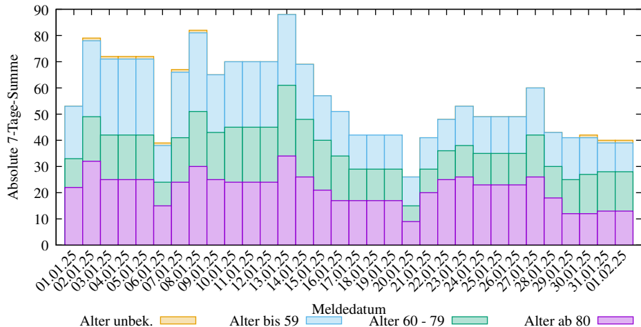
Abs. 7-Tage-Summen der neuen COVID-19 Infizierten in SK München (2025-03-09/2501, D. Lippold, https://covid19-de-stats.sourceforge.io/ Lizenz: CC BY-ND 4.0, Daten: Robert Koch-Institut (RKI), dl-de/by-2-0)
