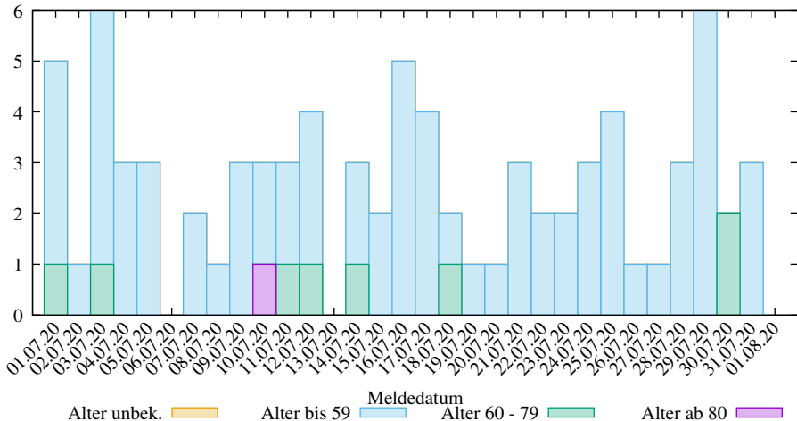
Einzelwerte der neuen COVID-19 Infizierten in LK München (2025-03-09/2007, D. Lippold, https://covid19-de-stats.sourceforge.io/ Lizenz: CC BY-ND 4.0, Daten: Robert Koch-Institut (RKI), dl-de/by-2-0)
