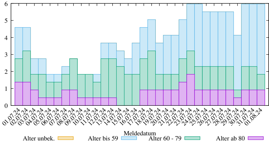
Rel. 7-Tage-Summe der neuen COVID-19 Infizierten in LK Rostock (2025-03-09/2407, D. Lippold, https://covid19-de-stats.sourceforge.io/ Lizenz: CC BY-ND 4.0, Daten: Robert Koch-Institut (RKI), dl-de/by-2-0)
