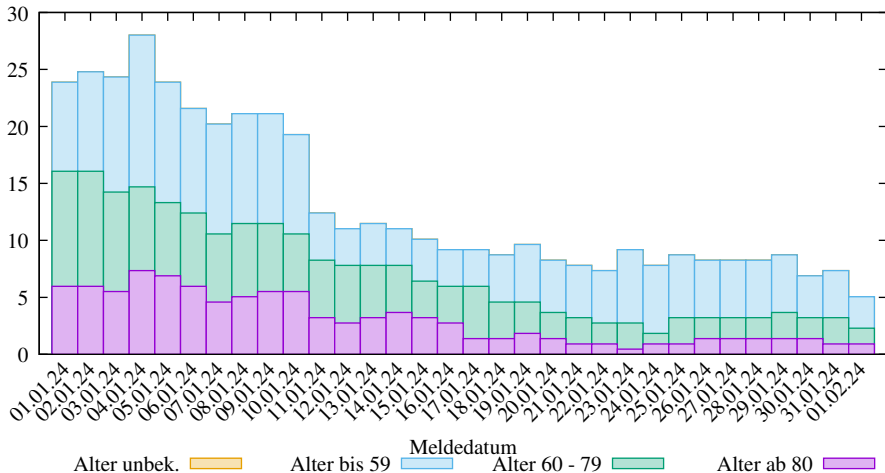
Rel. 7-Tage-Summe der neuen COVID-19 Infizierten in LK Rostock (2025-03-09/2401, D. Lippold, https://covid19-de-stats.sourceforge.io/ Lizenz: CC BY-ND 4.0, Daten: Robert Koch-Institut (RKI), dl-de/by-2-0)
