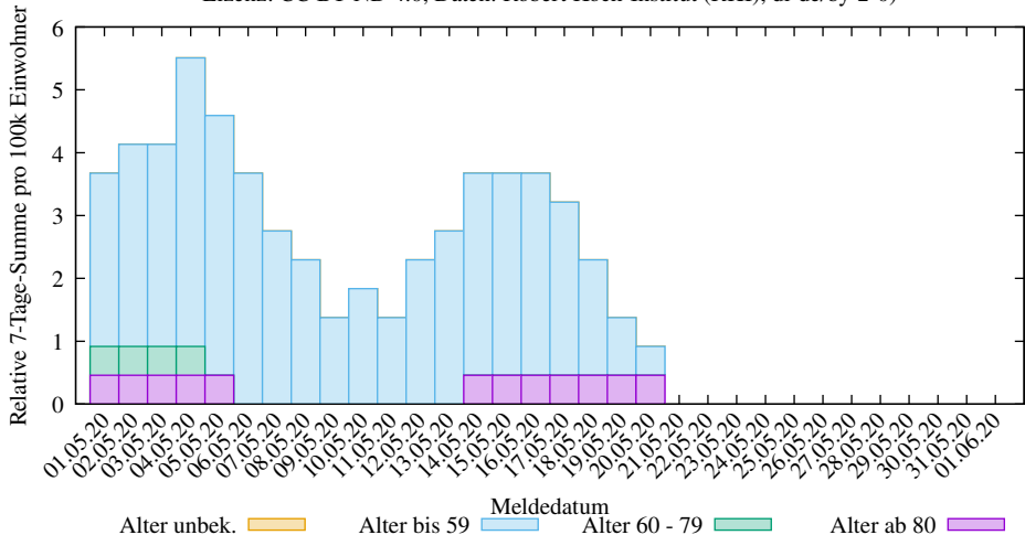
Rel. 7-Tage-Summe der neuen COVID-19 Infizierten in LK Rostock (2025-07-06/2005, D. Lippold, https://covid19-de-stats.sourceforge.io/ Lizenz: CC BY-ND 4.0, Daten: Robert Koch-Institut (RKI), dl-de/by-2-0)
