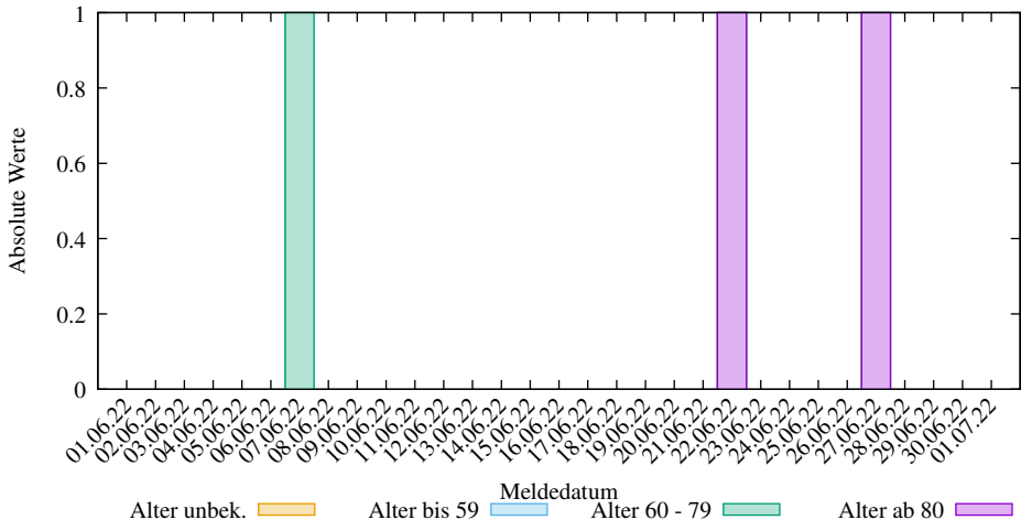
Einzelwerte der neuen COVID-19 Verstorbenen in LK Rostock (2025-03-09/2206, D. Lippold, https://covid19-de-stats.sourceforge.io/ Lizenz: CC BY-ND 4.0, Daten: Robert Koch-Institut (RKI), dl-de/by-2-0)
