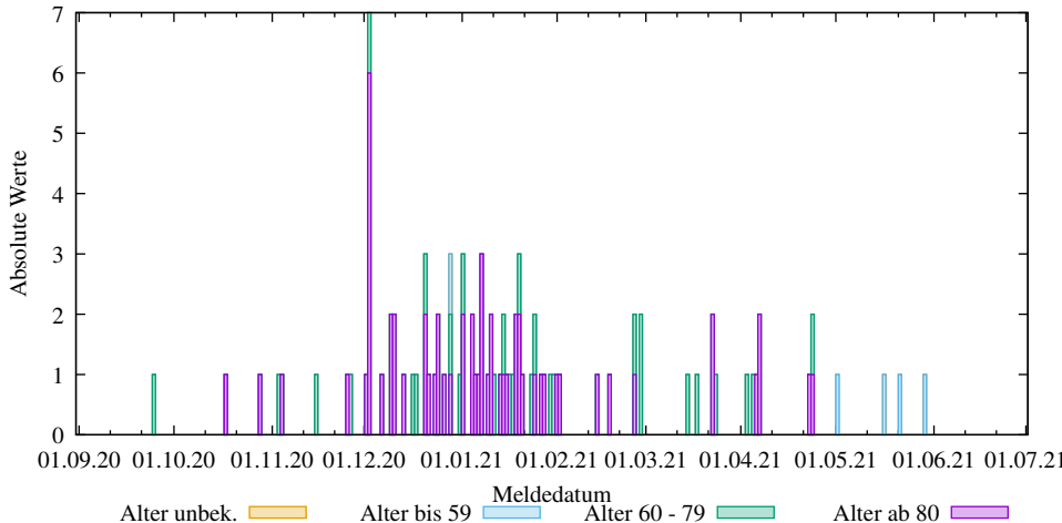
Einzelwerte der neuen COVID-19 Verstorbenen in SK Kiel (2025-03-09/Sp3, D. Lippold, https://covid19-de-stats.sourceforge.io/ Lizenz: CC BY-ND 4.0, Daten: Robert Koch-Institut (RKI), dl-de/by-2-0)
