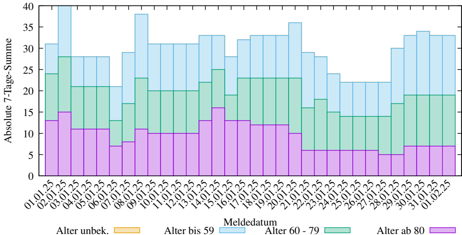
Abs. 7-Tage-Summen der neuen COVID-19 Infizierten in SK Köln (2025-03-09/2501, D. Lippold, https://covid19-de-stats.sourceforge.io/ Lizenz: CC BY-ND 4.0, Daten: Robert Koch-Institut (RKI), dl-de/by-2-0)
