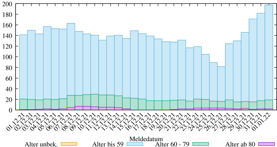
Rel. 7-Tage-Summe der neuen COVID-19 Infizierten in LK Steinburg (2025-03-09/2112, D. Lippold, https://covid19-de-stats.sourceforge.io/ Lizenz: CC BY-ND 4.0, Daten: Robert Koch-Institut (RKI), dl-de/by-2-0)
