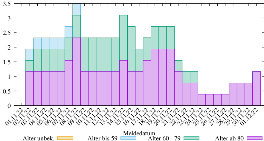
Rel. 7-Tage-Summe der neuen COVID-19 Verstorbenen in LK Heinsberg (2025-03-09/2211, D. Lippold, https://covid19-de-stats.sourceforge.io/ ) Lizenz: CC BY-ND 4.0, Daten: Robert Koch-Institut (RKI), dl-de/by-2-0)
