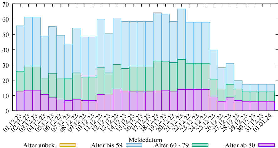
Rel. 7-Tage-Summe der neuen COVID-19 Infizierten in SK Rostock (2025-03-09/2312, D. Lippold, https://covid19-de-stats.sourceforge.io/ Lizenz: CC BY-ND 4.0, Daten: Robert Koch-Institut (RKI), dl-de/by-2-0)
