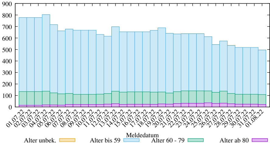
Rel. 7-Tage-Summe der neuen COVID-19 Infizierten in SK Rostock (2025-03-09/2207, D. Lippold, https://covid19-de-stats.sourceforge.io/ ) Lizenz: CC BY-ND 4.0, Daten: Robert Koch-Institut (RKI), dl-de/by-2-0)
