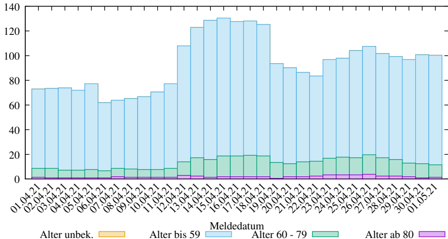
Rel. 7-Tage-Summe der neuen COVID-19 Infizierten in SK Rostock (2025-03-09/2104, D. Lippold, https://covid19-de-stats.sourceforge.io/ Lizenz: CC BY-ND 4.0, Daten: Robert Koch-Institut (RKI), dl-de/by-2-0)
