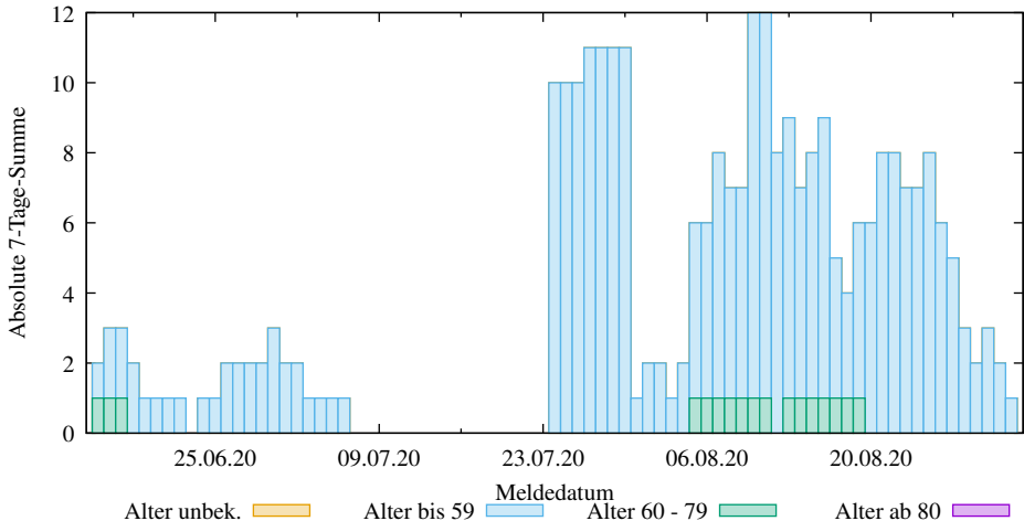
Abs. 7-Tage-Summen der neuen COVID-19 Infizierten in SK Rostock (2025-03-09/Sp2, D. Lippold, https://covid19-de-stats.sourceforge.io/ Lizenz: CC BY-ND 4.0, Daten: Robert Koch-Institut (RKI), dl-de/by-2-0)
