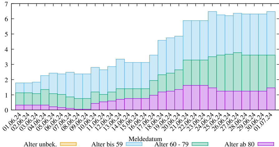
Rel. 7-Tage-Summe der neuen COVID-19 Infizierten in SK Hamburg (2025-03-09/2406, D. Lippold, https://covid19-de-stats.sourceforge.io/ Lizenz: CC BY-ND 4.0, Daten: Robert Koch-Institut (RKI), dl-de/by-2-0)
