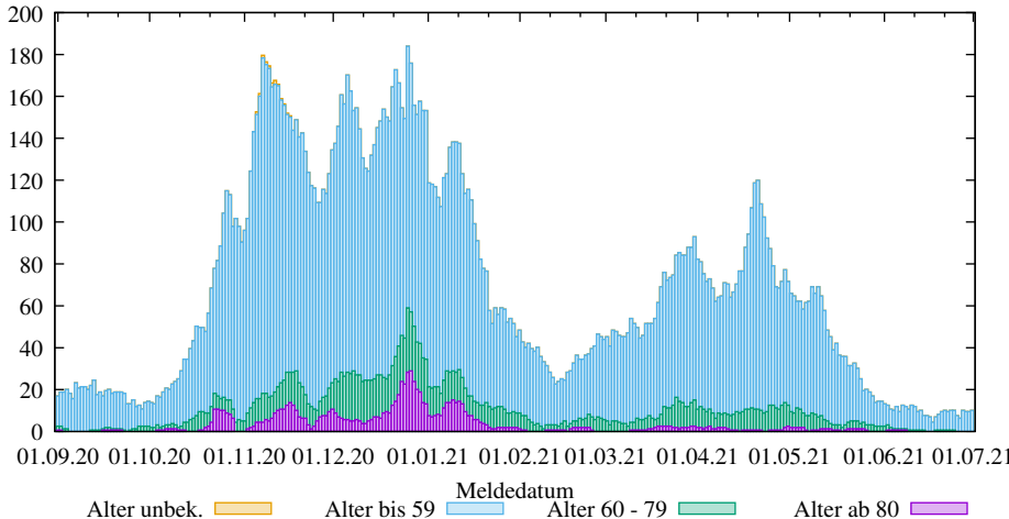
Rel. 7-Tage-Summe der neuen COVID-19 Infizierten in SK Heidelberg (2025-03-09/Sp3, D. Lippold, https://covid19-de-stats.sourceforge.io/ ) Lizenz: CC BY-ND 4.0, Daten: Robert Koch-Institut (RKI), dl-de/by-2-0)
