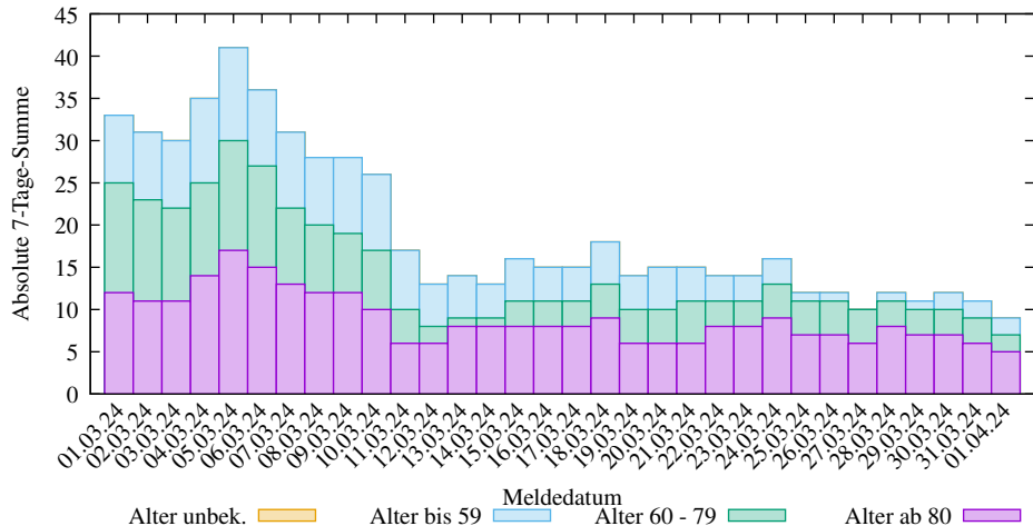
Abs. 7-Tage-Summen der neuen COVID-19 Infizierten in Region Hannover (2025-03-09/2403, D. Lippold, https://covid19-de-stats.sourceforge.io/ Lizenz: CC BY-ND 4.0, Daten: Robert Koch-Institut (RKI), dl-de/by-2-0)
