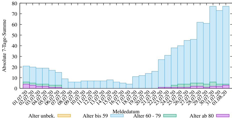
Abs. 7-Tage-Summen der neuen COVID-19 Infizierten in Region Hannover (2025-03-09/2007, D. Lippold, https://covid19-de-stats.sourceforge.io/ Lizenz: CC BY-ND 4.0, Daten: Robert Koch-Institut (RKI), dl-de/by-2-0)
