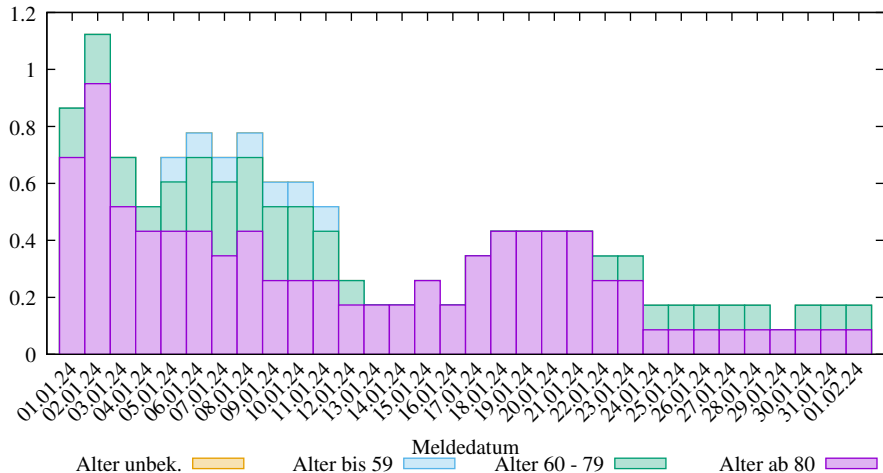
Rel. 7-Tage-Summe der neuen COVID-19 Verstorbenen in Region Hannover (2025-03-09/2401, D. Lippold, https://covid19-de-stats.sourceforge.io/ Lizenz: CC BY-ND 4.0, Daten: Robert Koch-Institut (RKI), dl-de/by-2-0)
