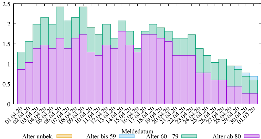
Rel. 7-Tage-Summe der neuen COVID-19 Verstorbenen in Region Hannover (2025-03-09/2004, D. Lippold, https://covid19-de-stats.sourceforge.io/ Lizenz: CC BY-ND 4.0, Daten: Robert Koch-Institut (RKI), dl-de/by-2-0)
