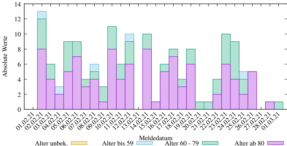
Einzelwerte der neuen COVID-19 Verstorbenen in Region Hannover (2025-03-09/2102, D. Lippold, https://covid19-de-stats.sourceforge.io/ Lizenz: CC BY-ND 4.0, Daten: Robert Koch-Institut (RKI), dl-de/by-2-0)
