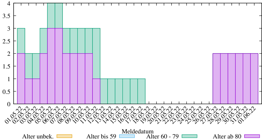
Abs. 7-Tage-Summen der neuen COVID-19 Verstorbenen in LK Gütersloh (2025-03-09/2205, D. Lippold, https://covid19-de-stats.sourceforge.io/ Lizenz: CC BY-ND 4.0, Daten: Robert Koch-Institut (RKI), dl-de/by-2-0)
