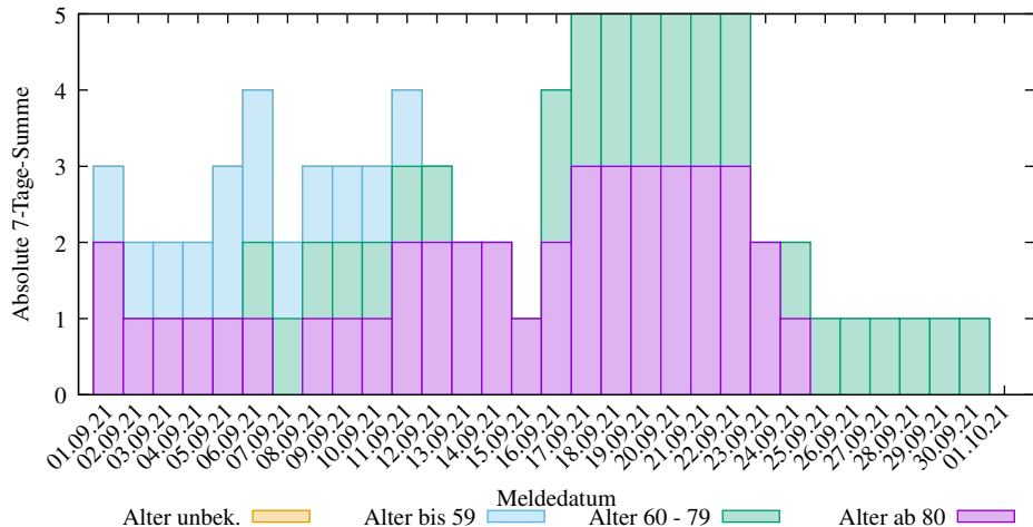
Abs. 7-Tage-Summen der neuen COVID-19 Verstorbenen in LK Gütersloh (2025-03-09/2109, D. Lippold, https://covid19-de-stats.sourceforge.io/ Lizenz: CC BY-ND 4.0, Daten: Robert Koch-Institut (RKI), dl-de/by-2-0)
