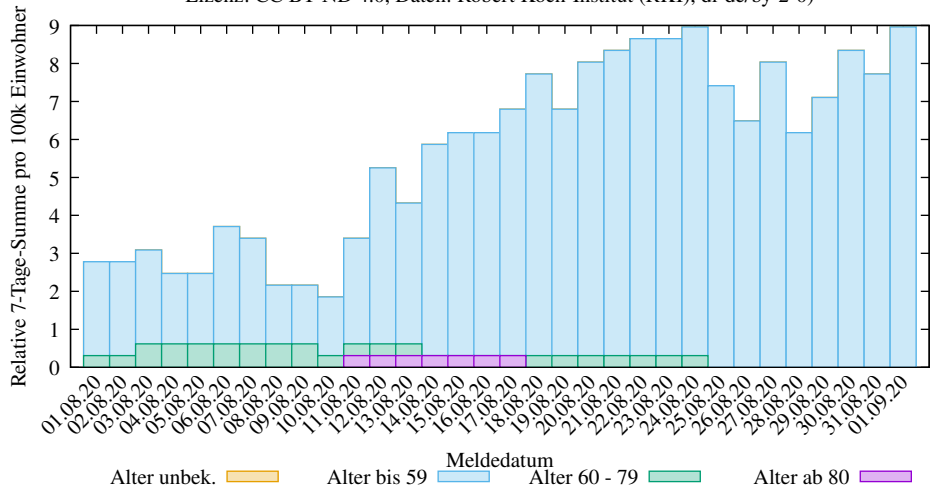
Rel. 7-Tage-Summe der neuen COVID-19 Infizierten in LK Göttingen (2025-03-09/2008, D. Lippold, https://covid19-de-stats.sourceforge.io/ Lizenz: CC BY-ND 4.0, Daten: Robert Koch-Institut (RKI), dl-de/by-2-0)
