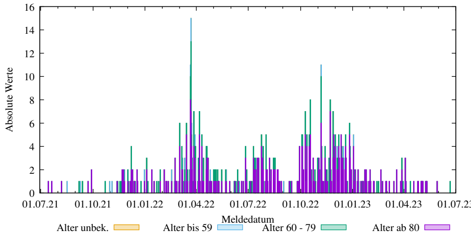
Einzelwerte der neuen COVID-19 Verstorbenen in SK Braunschweig (2025-03-09/Sp4, D. Lippold, https://covid19-de-stats.sourceforge.io/ Lizenz: CC BY-ND 4.0, Daten: Robert Koch-Institut (RKI), dl-de/by-2-0)
