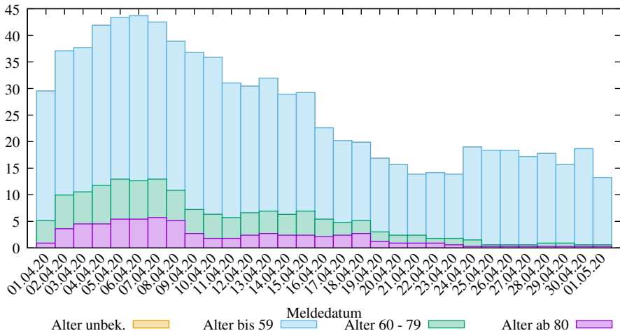
Rel. 7-Tage-Summe der neuen COVID-19 Infizierten in SK Bonn (2025-03-09/2004, D. Lippold, https://covid19-de-stats.sourceforge.io/ Lizenz: CC BY-ND 4.0, Daten: Robert Koch-Institut (RKI), dl-de/by-2-0)
