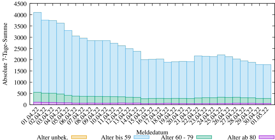
Abs. 7-Tage-Summen der neuen COVID-19 Infizierten in SK Bonn (2025-03-09/2204, D. Lippold, https://covid19-de-stats.sourceforge.io/ Lizenz: CC BY-ND 4.0, Daten: Robert Koch-Institut (RKI), dl-de/by-2-0)
