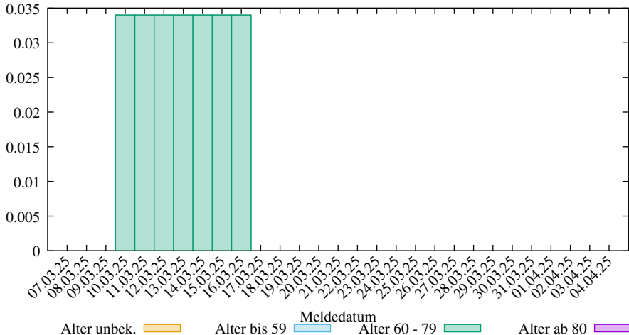
Rel. 7-Tage-Summe der neuen COVID-19 Verstorbenen in Schleswig-Holstein (2025-04-26/Limit, D. Lippold, https://covid19-de-stats.sourceforge.io/ Lizenz: CC BY-ND 4.0, Daten: Robert Koch-Institut (RKI), dl-de/by-2-0)
