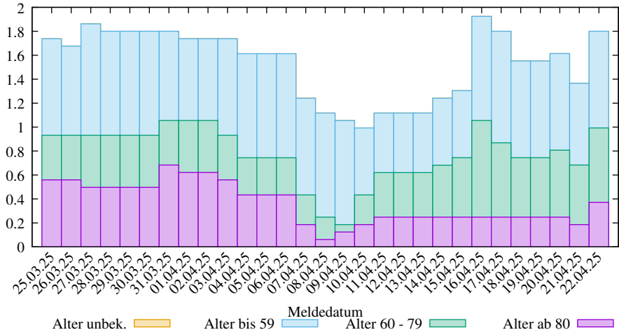
Rel. 7-Tage-Summe der neuen COVID-19 Infizierten in Meckl.-Vorpom. (2025-04-26/Limit, D. Lippold, https://covid19-de-stats.sourceforge.io/ Lizenz: CC BY-ND 4.0, Daten: Robert Koch-Institut (RKI), dl-de/by-2-0)
