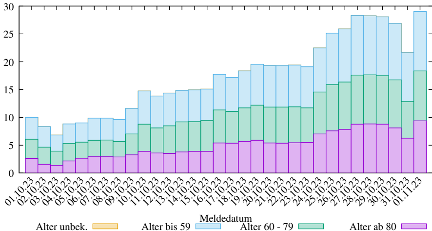
Rel. 7-Tage-Summe der neuen COVID-19 Infizierten in Thüringen (2025-03-09/2310, D. Lippold, https://covid19-de-stats.sourceforge.io/ Lizenz: CC BY-ND 4.0, Daten: Robert Koch-Institut (RKI), dl-de/by-2-0)
