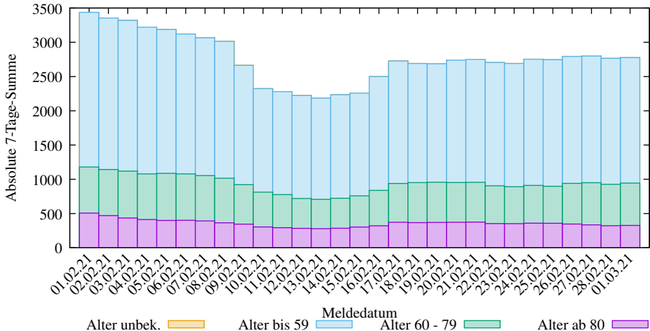
Abs. 7-Tage-Summen der neuen COVID-19 Infizierten in Thüringen (2025-03-09/2102, D. Lippold, https://covid19-de-stats.sourceforge.io/ Lizenz: CC BY-ND 4.0, Daten: Robert Koch-Institut (RKI), dl-de/by-2-0)
