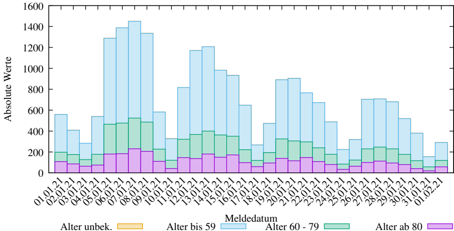
Einzelwerte der neuen COVID-19 Infizierten in Thüringen (2025-03-09/2101, D. Lippold, https://covid19-de-stats.sourceforge.io/ Lizenz: CC BY-ND 4.0, Daten: Robert Koch-Institut (RKI), dl-de/by-2-0)
