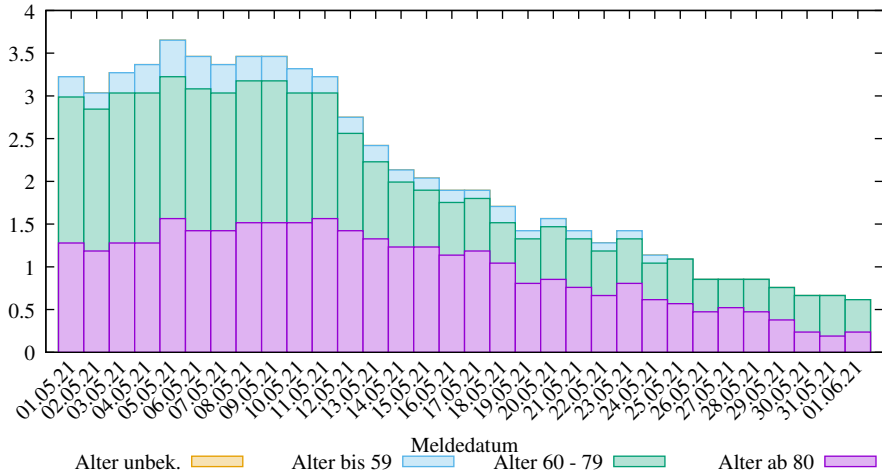
Rel. 7-Tage-Summe der neuen COVID-19 Verstorbenen in Thüringen (2025-03-09/2105, D. Lippold, https://covid19-de-stats.sourceforge.io/ Lizenz: CC BY-ND 4.0, Daten: Robert Koch-Institut (RKI), dl-de/by-2-0)
