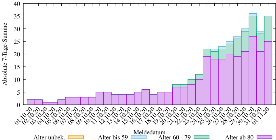
Abs. 7-Tage-Summen der neuen COVID-19 Verstorbenen in Thüringen (2025-03-09/2010, D. Lippold, https://covid19-de-stats.sourceforge.io/ Lizenz: CC BY-ND 4.0, Daten: Robert Koch-Institut (RKI), dl-de/by-2-0)
