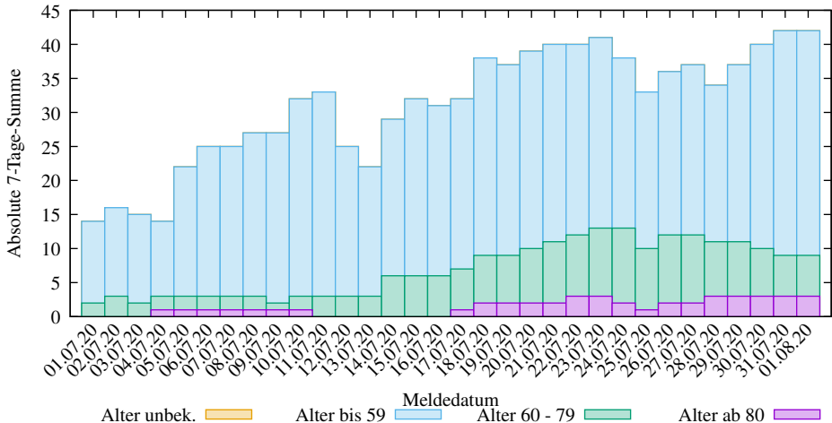
Abs. 7-Tage-Summen der neuen COVID-19 Infizierten in Sachsen-Anhalt (2025-03-09/2007, D. Lippold, https://covid19-de-stats.sourceforge.io/ Lizenz: CC BY-ND 4.0, Daten: Robert Koch-Institut (RKI), dl-de/by-2-0)
