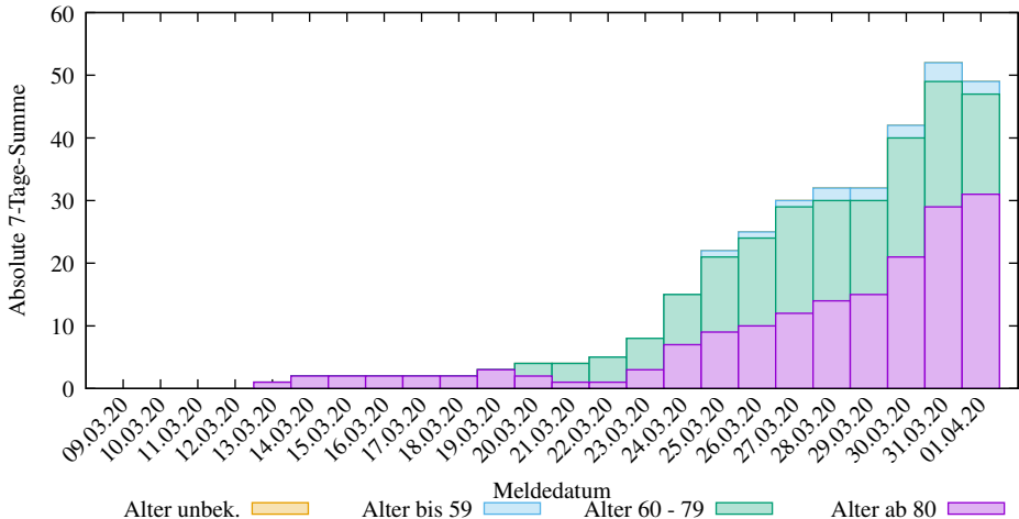
Abs. 7-Tage-Summen der neuen COVID-19 Verstorbenen in Sachsen (2025-03-09/2003, D. Lippold, https://covid19-de-stats.sourceforge.io/ Lizenz: CC BY-ND 4.0, Daten: Robert Koch-Institut (RKI), dl-de/by-2-0)
