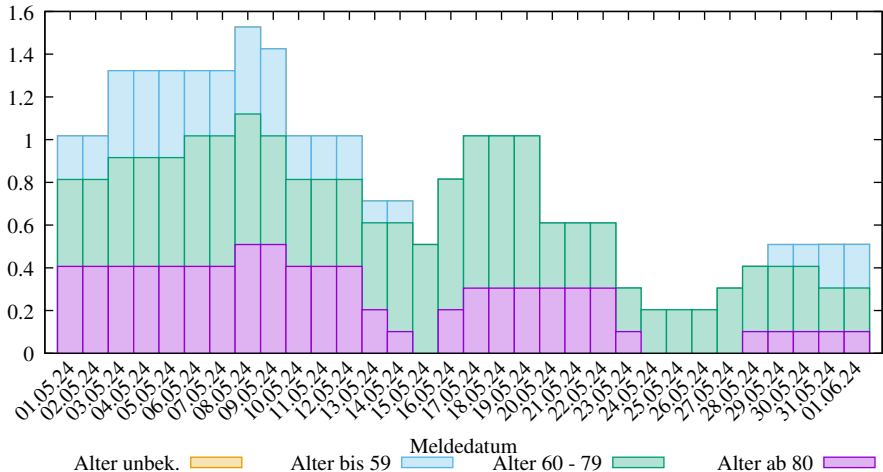
Rel. 7-Tage-Summe der neuen COVID-19 Infizierten in Saarland (2025-03-09/2405, D. Lippold, https://covid19-de-stats.sourceforge.io/ Lizenz: CC BY-ND 4.0, Daten: Robert Koch-Institut (RKI), dl-de/by-2-0)
