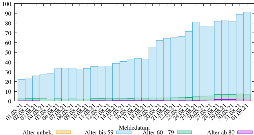
Rel. 7-Tage-Summe der neuen COVID-19 Infizierten in Saarland (2025-03-09/2108, D. Lippold, https://covid19-de-stats.sourceforge.io/ Lizenz: CC BY-ND 4.0, Daten: Robert Koch-Institut (RKI), dl-de/by-2-0)
