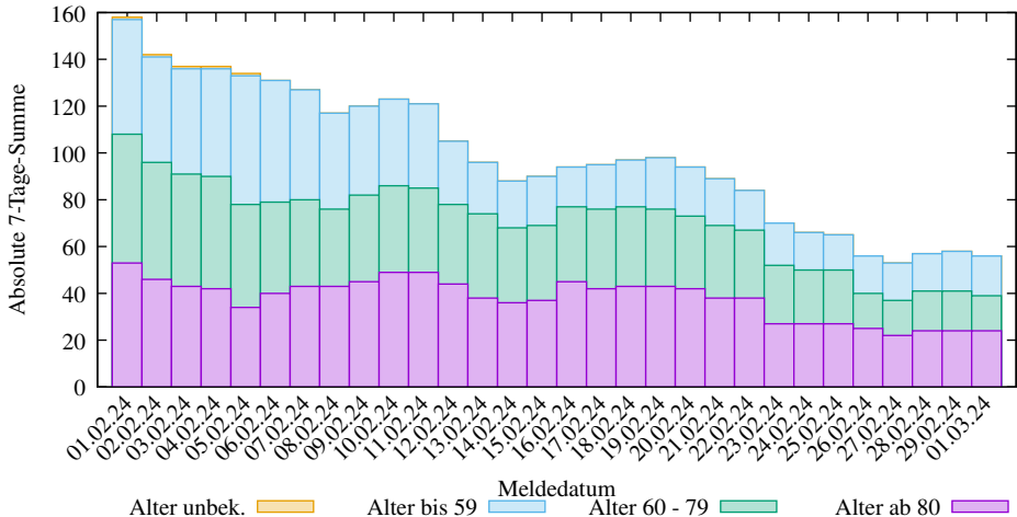
Abs. 7-Tage-Summen der neuen COVID-19 Infizierten in Schleswig-Holstein (2025-03-09/2402, D. Lippold, https://covid19-de-stats.sourceforge.io/ Lizenz: CC BY-ND 4.0, Daten: Robert Koch-Institut (RKI), dl-de/by-2-0)
