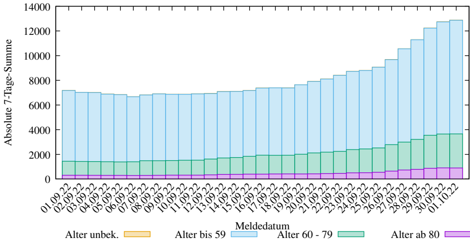
Abs. 7-Tage-Summen der neuen COVID-19 Infizierten in Schleswig-Holstein (2025-03-09/2209, D. Lippold, https://covid19-de-stats.sourceforge.io/ Lizenz: CC BY-ND 4.0, Daten: Robert Koch-Institut (RKI), dl-de/by-2-0)
