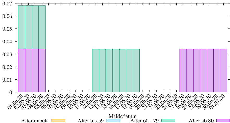
Rel. 7-Tage-Summe der neuen COVID-19 Verstorbenen in Schleswig-Holstein (2025-03-09/2006, D. Lippold, https://covid19-de-stats.sourceforge.io/ Lizenz: CC BY-ND 4.0, Daten: Robert Koch-Institut (RKI), dl-de/by-2-0)
