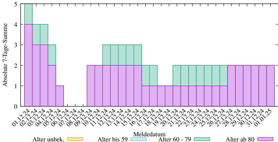
Abs. 7-Tage-Summen der neuen COVID-19 Verstorbenen in Schleswig-Holstein (2025-03-09/2412, D. Lippold, https://covid19-de-stats.sourceforge.io/ Lizenz: CC BY-ND 4.0, Daten: Robert Koch-Institut (RKI), dl-de/by-2-0)
