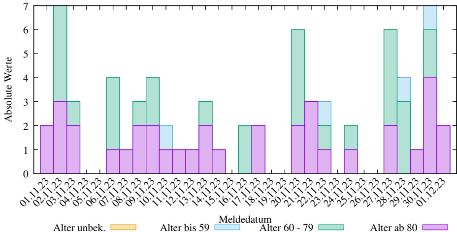
Einzelwerte der neuen COVID-19 Verstorbenen in Schleswig-Holstein (2025-03-09/2311, D. Lippold, https://covid19-de-stats.sourceforge.io/ Lizenz: CC BY-ND 4.0, Daten: Robert Koch-Institut (RKI), dl-de/by-2-0)
