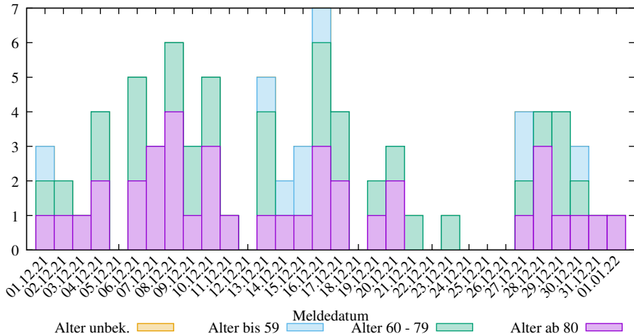
Einzelwerte der neuen COVID-19 Verstorbenen in Schleswig-Holstein (2025-03-09/2112, D. Lippold, https://covid19-de-stats.sourceforge.io/ Lizenz: CC BY-ND 4.0, Daten: Robert Koch-Institut (RKI), dl-de/by-2-0)
