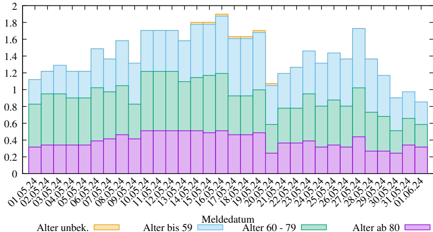
Rel. 7-Tage-Summe der neuen COVID-19 Infizierten in Rheinland-Pfalz (2025-03-09/2405, D. Lippold, https://covid19-de-stats.sourceforge.io/ Lizenz: CC BY-ND 4.0, Daten: Robert Koch-Institut (RKI), dl-de/by-2-0)
